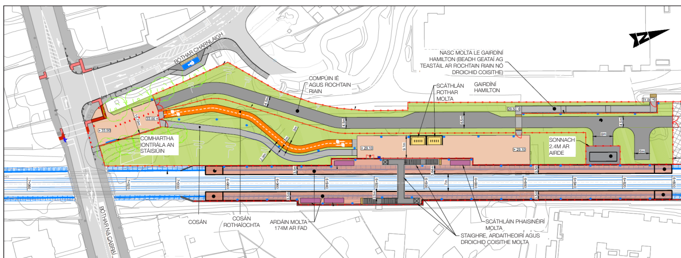
Leagan Amach Coincheap Stáisiún na Cabraí
