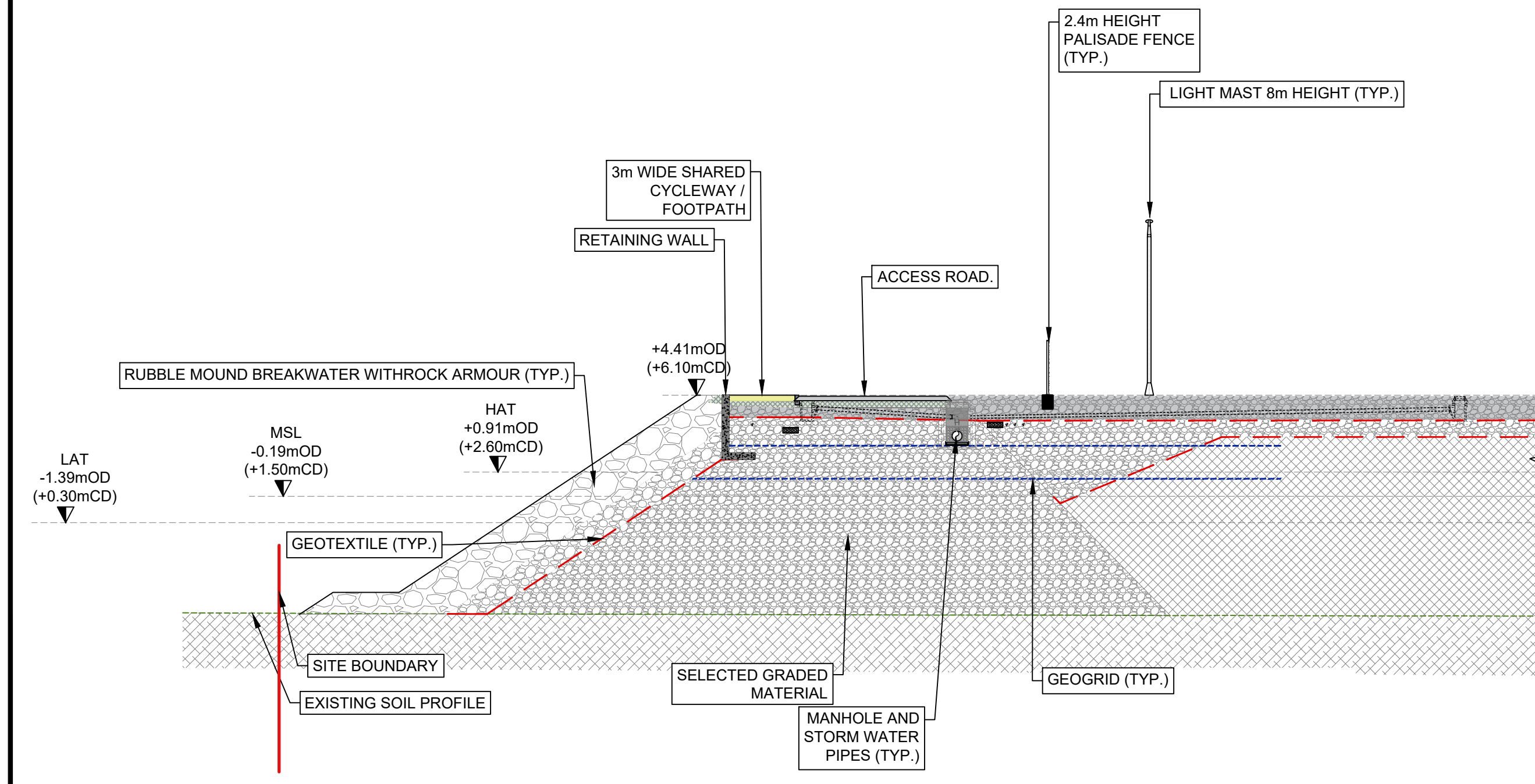
SECTION E-E-VIEW 9 SCALE: 1:200
